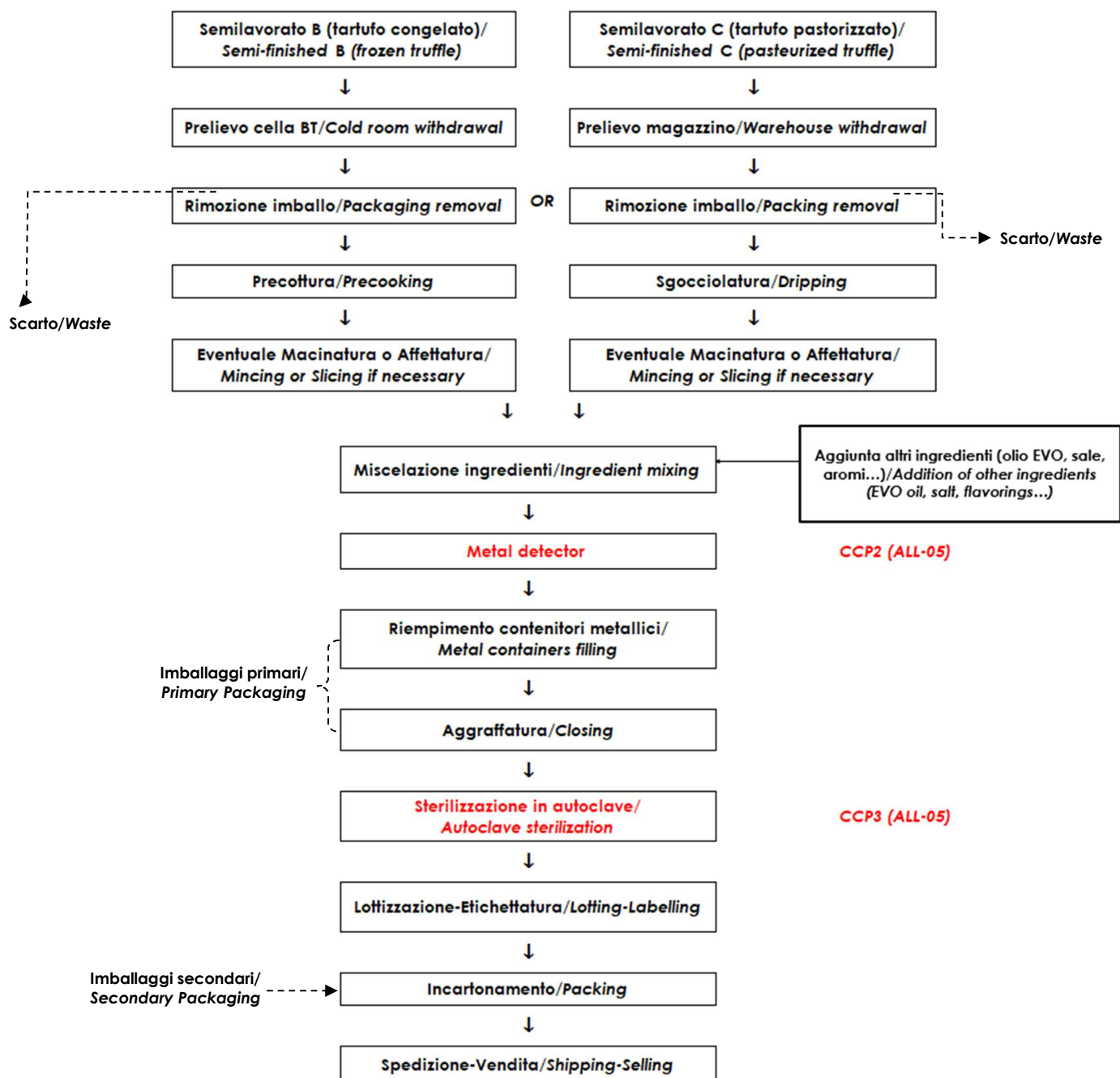
DIAGRAMMA DI FLUSSO: LAVORAZIONE DI PRODOTTI FINITI INDUSTRIALI FLOW CHART: PROCESSING OF INDUSTRIAL FINISHED PRODUCTS
